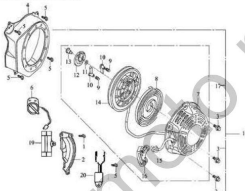
E-10 反冲起动器部件 RECOIL STARTER
